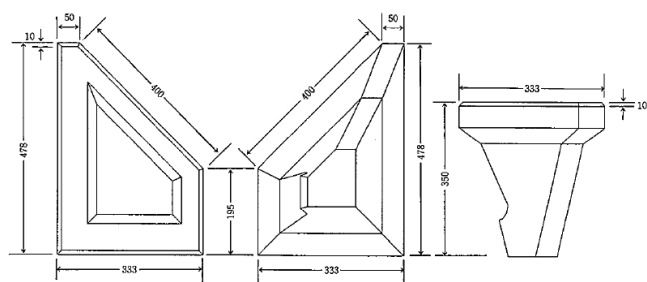
D (隅角) 型 (図は左大)
