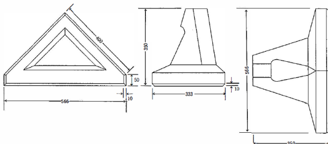
E (隅角) 型 (図は右小)
