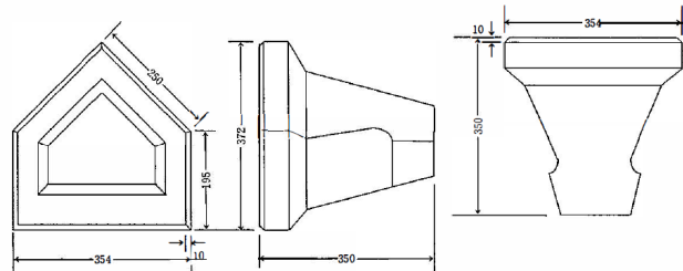
B (基礎天端) 型
