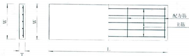
寸法及び配筋表
