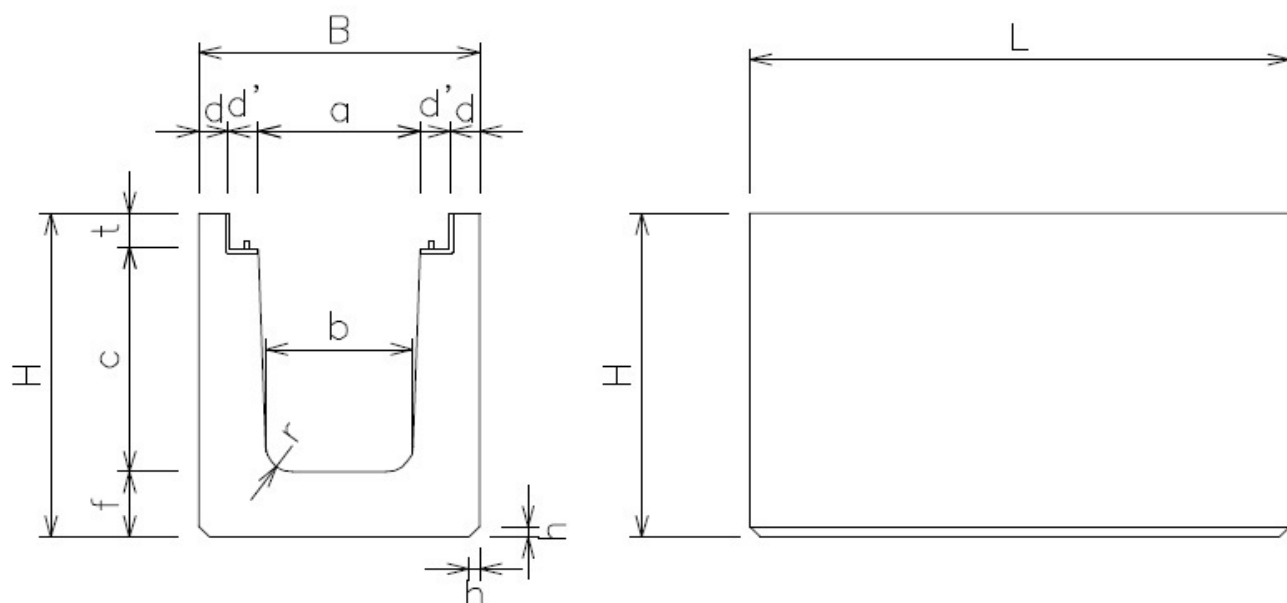
製品寸法表
